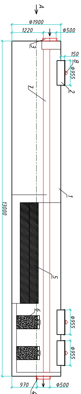
Разрез 1-1
